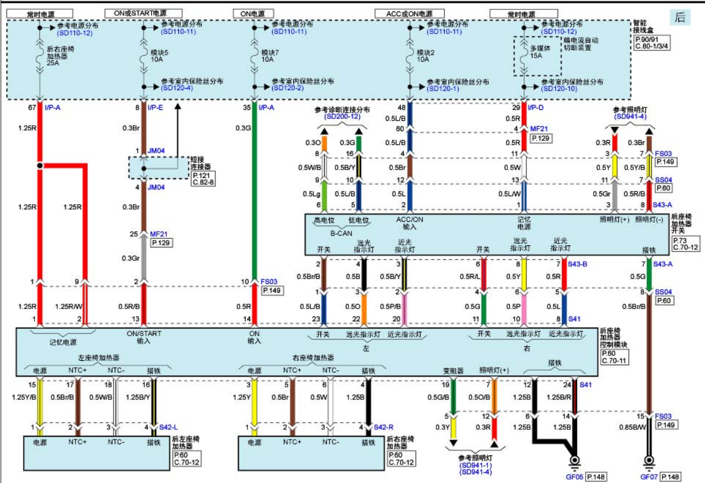
座椅加热器系统(3)
